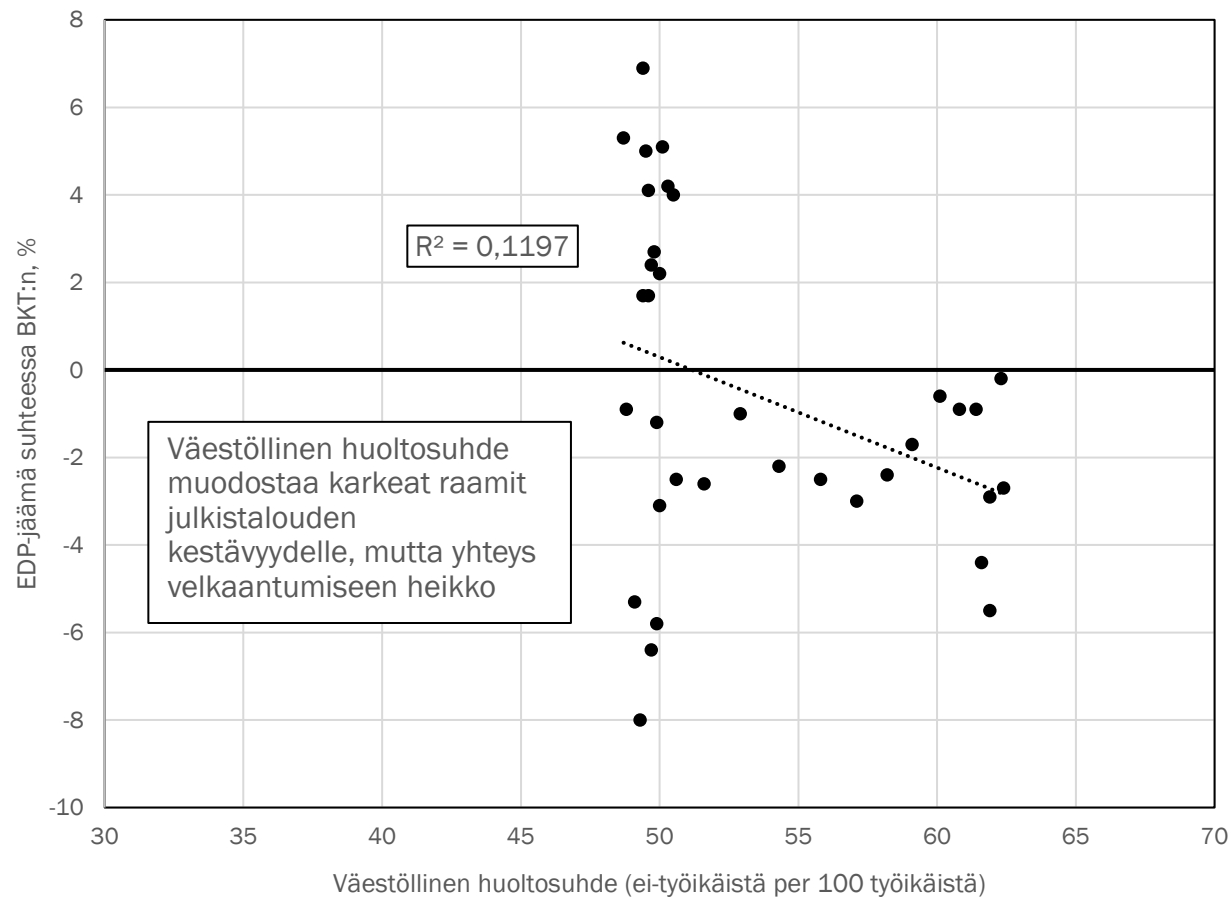
Velkaantumisen ja väestöllisen huoltosuhteen yhteys ('90-'24)
